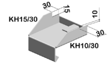
Spez. Klinkung Bord KH15/30
