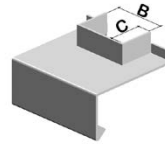
Pfeilerausschnitt mit Stehbord 3-seitig
