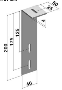
Langlöcher 6.5 x 26 mm
