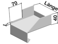
Stehbord St40-7/70
